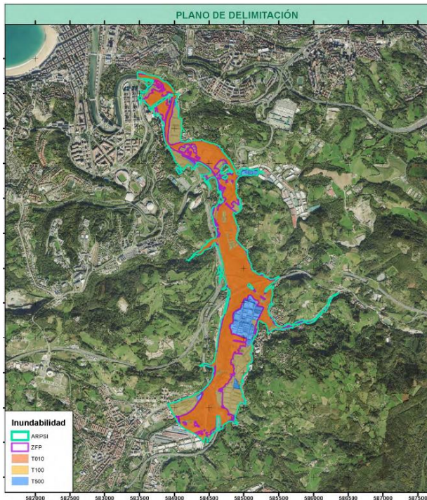
Irudia 16 Uholde arriskua Astigarragan Iturria: URA
